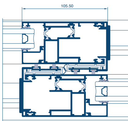
Sección central
