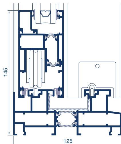
Sección lateral
